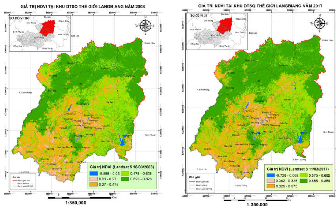
Hình 3. Giá trị chỉ số NDVI tính toán theo Landsat 5 (18/03/2008); Landsat 8 (11/03/2017)
